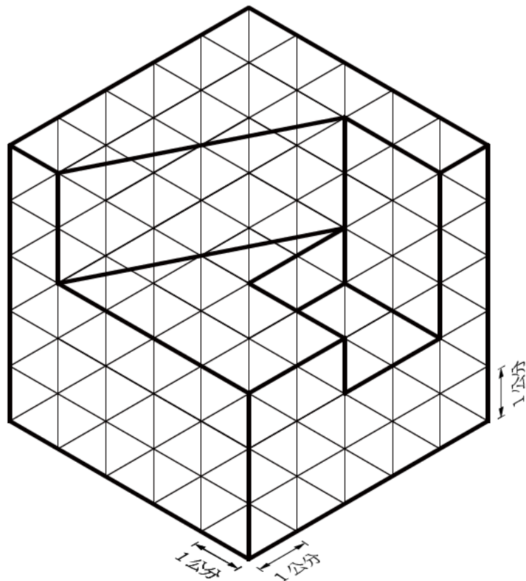
圖(一) 物體之等角圖
