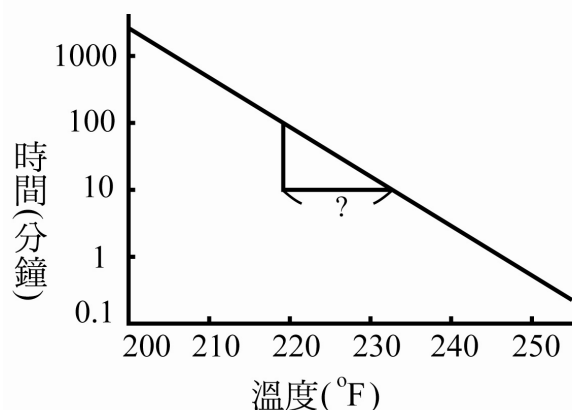
圖(一)細菌的孢子加熱致死時間曲線
